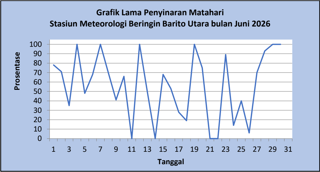
Gambar 4 Grafik Penyinaran Matahari harian Muara Teweh Bulan Juni 2026
