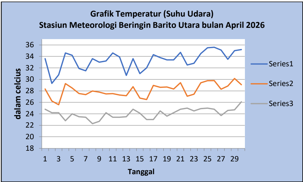
Gambar 2 Grafik Suhu Udara Bulan April 2026
