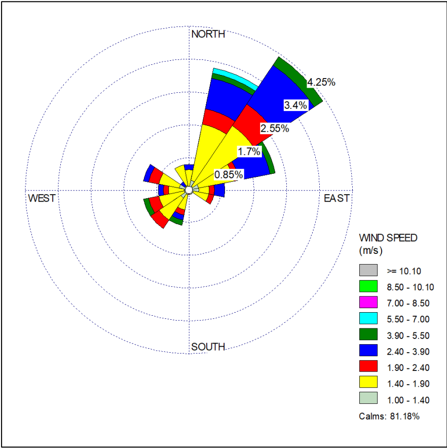
Gambar 9 Windrose Wilayah Muara Teweh Bulan April 2026
