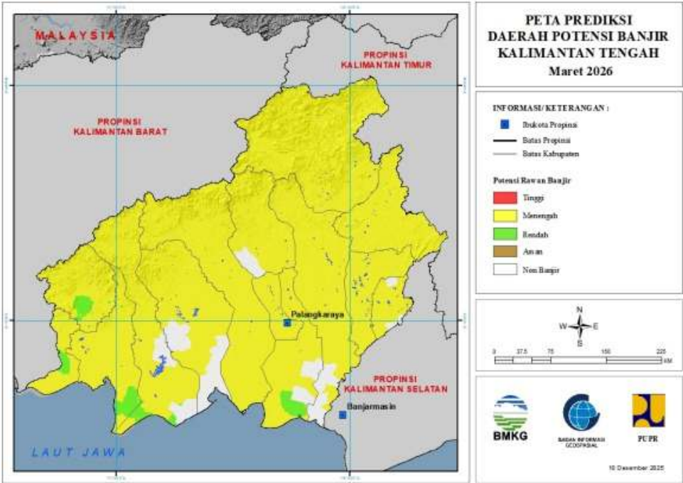
Gambar 19 Peta Prakiraan Daerah Potensi Banjir Juli 2026
