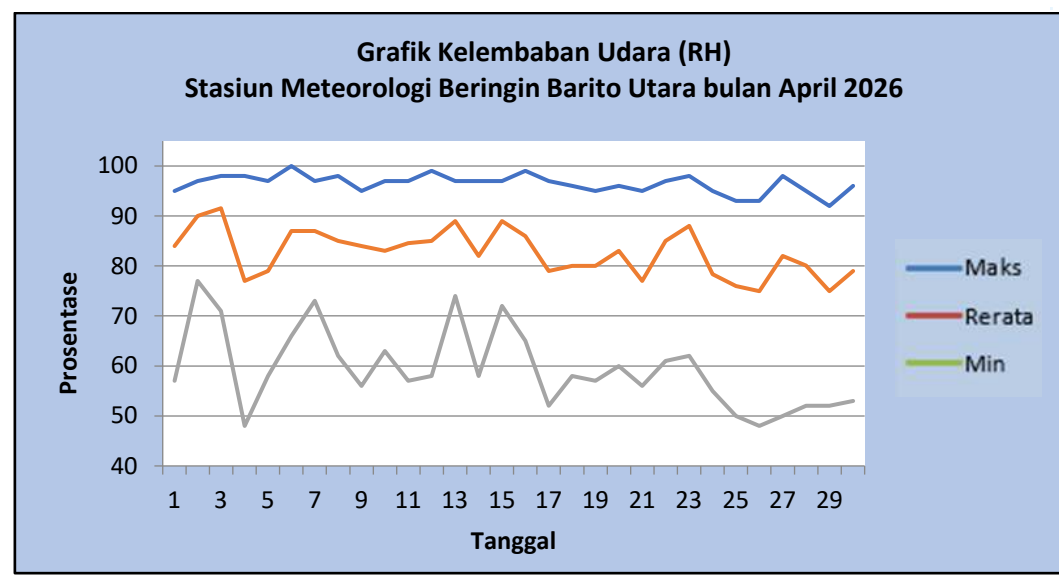
Gambar 3 Grafik Kelembaban Udara Muara Teweh Bulan April 2026
