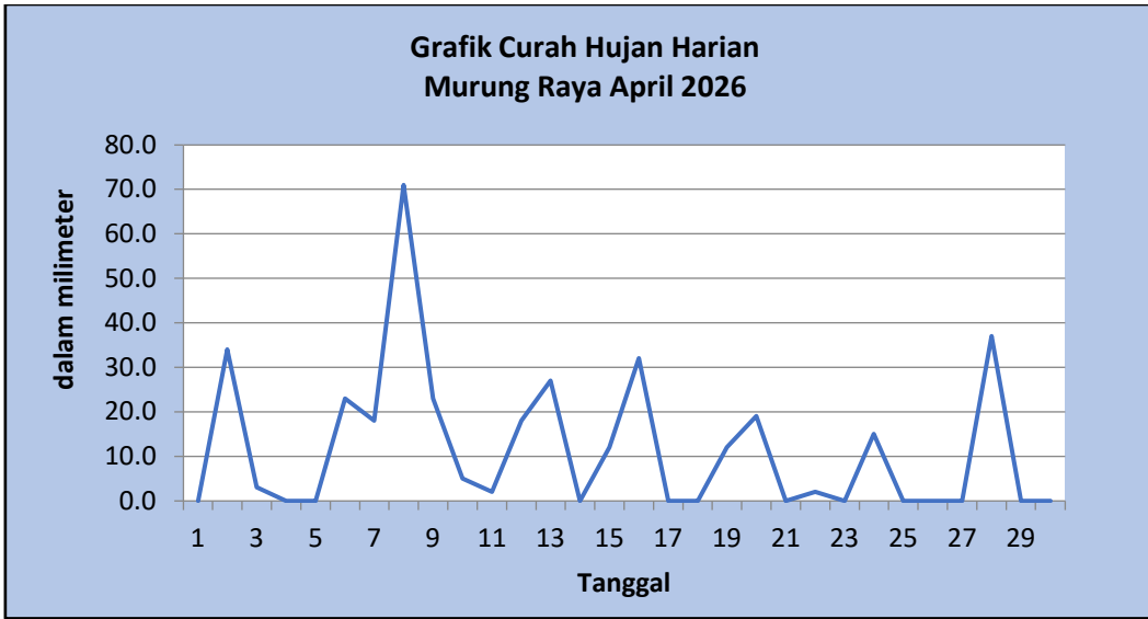
Gambar 7 Grafik Curah Hujan Murung Raya Bulan April 2026
