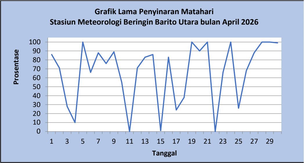
Gambar 4 Grafik Penyinaran Matahari harian Muara Teweh Bulan April 2026
