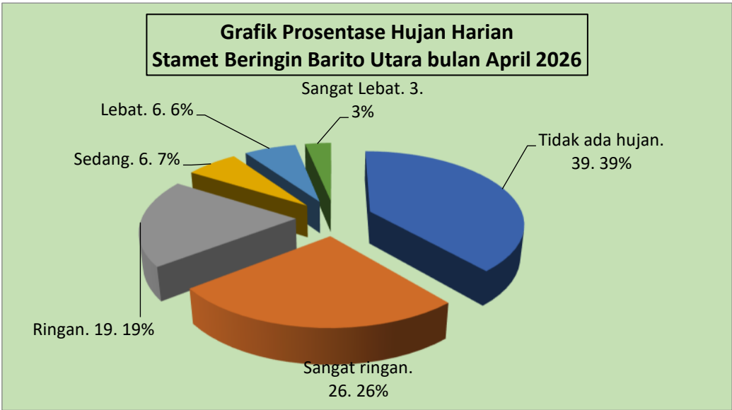
Gambar 12 Grafik Intensitas Hujan Harian Muara Teweh Bulan April 2026
