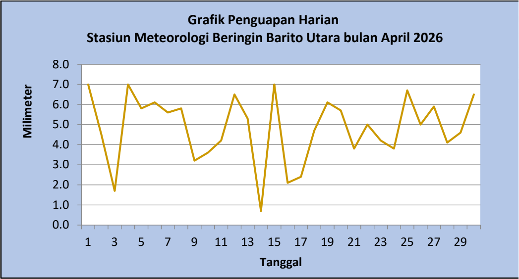
Gambar 5 Grafik Penguapan Harian Muara Teweh Bulan April 2026
