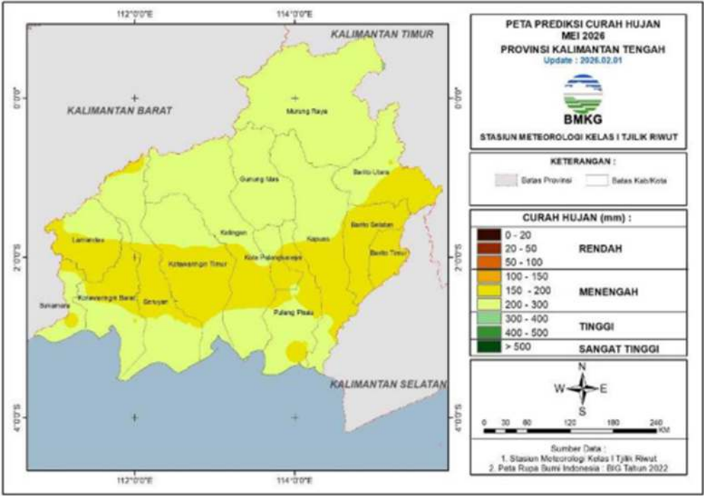
Gambar 14 Peta Prakiraan Curah Hujan Bulan Mei 2026
