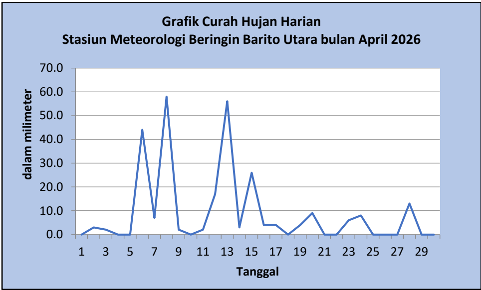
Gambar 6 Grafik Curah Hujan di Muara Teweh Bulan April 2026
