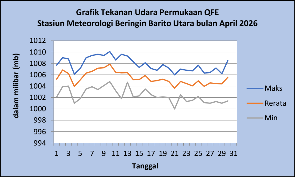
Gambar 1 Tekanan Udara Harian Muara Teweh Bulan April 2026
