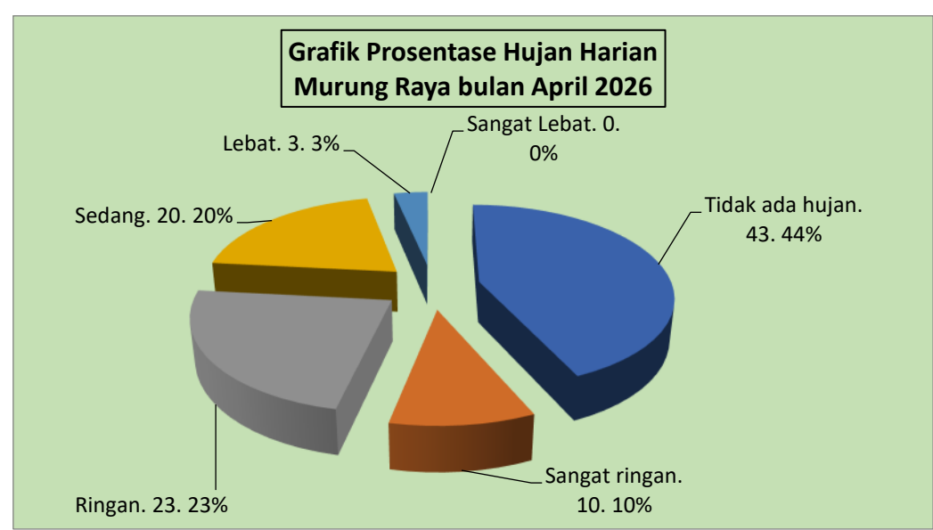
Gambar 13 Grafik Intensitas Hujan Harian Murung Raya Bulan April 2026
